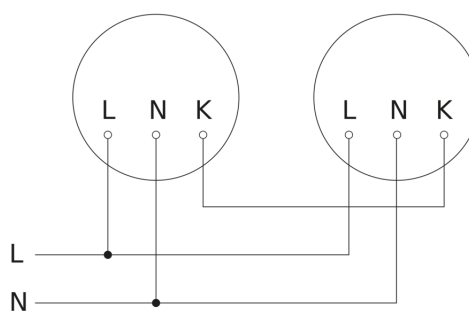
Diagrama electrónico interconexión maestro-maestro
